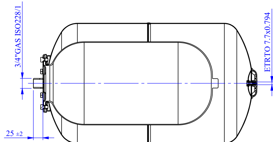
SEZIONE A-A
